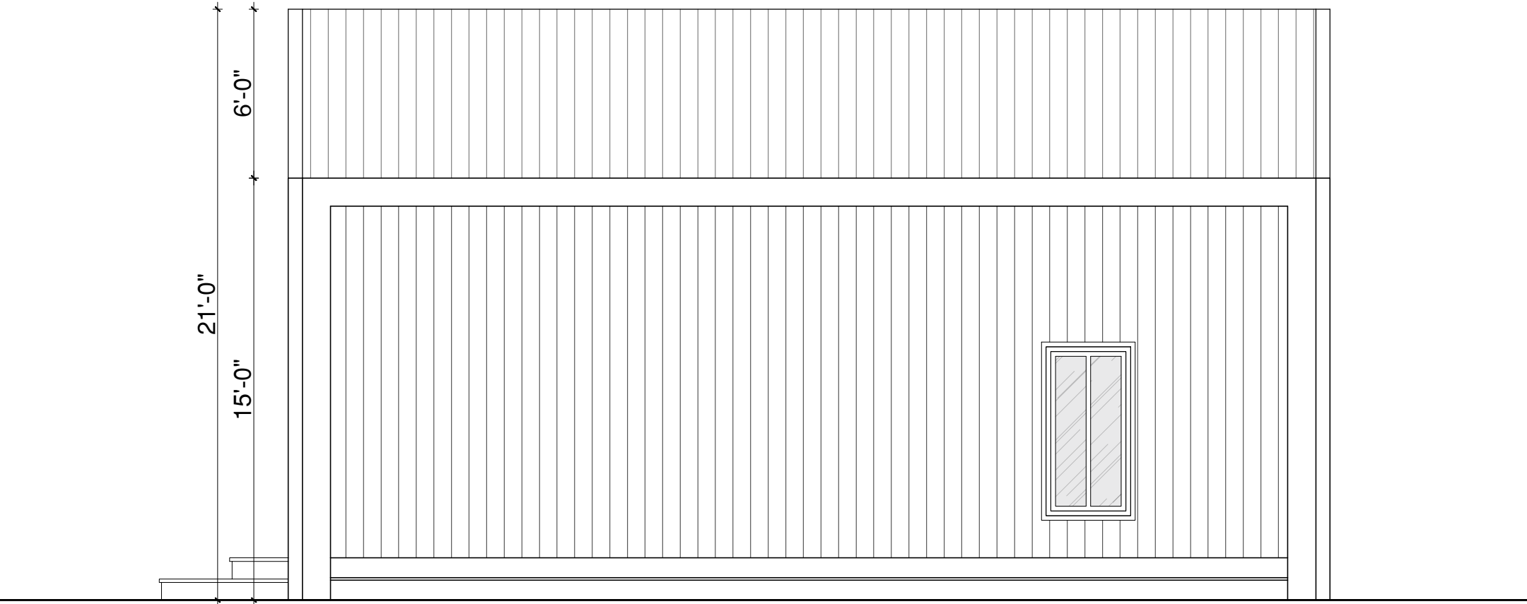
RIGHT ELEVATION
